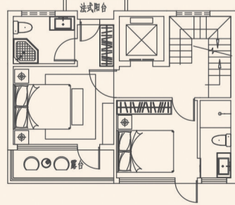
【三层平面图】 本层面积约45m 2
