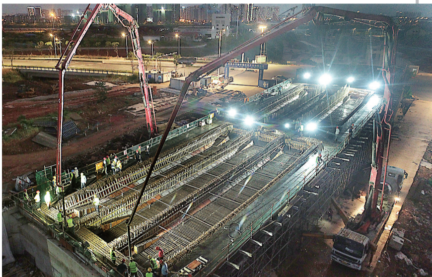
浇筑施工现场。通讯员供图
