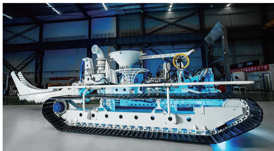
▲中车时代电气旗下SMD公司打造的智能水下挖沟铺缆机 受访企业供图
