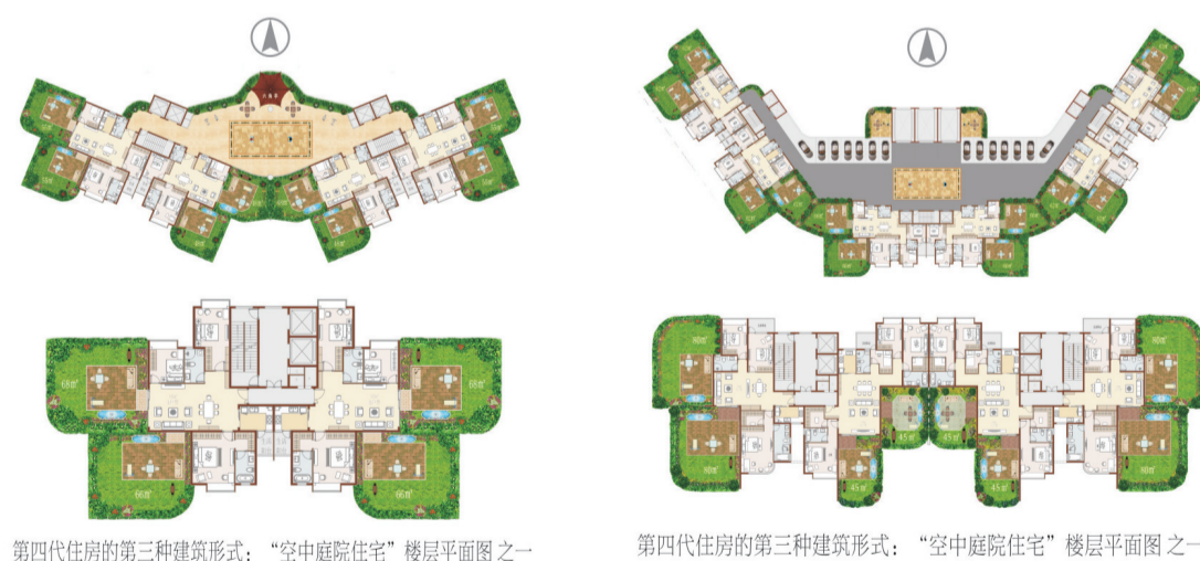
第四代住房的第三种建筑形式：“空中庭院住宅”楼层平面图之一
