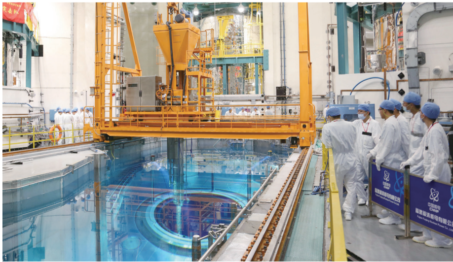
9月4日,“华龙一号”全球首堆中核集团福清核电5号机组,第1组燃料组件顺利入堆。新华社发(胡杰摄)
