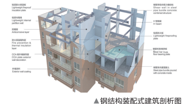
▲钢结构装配式建筑剖析图
