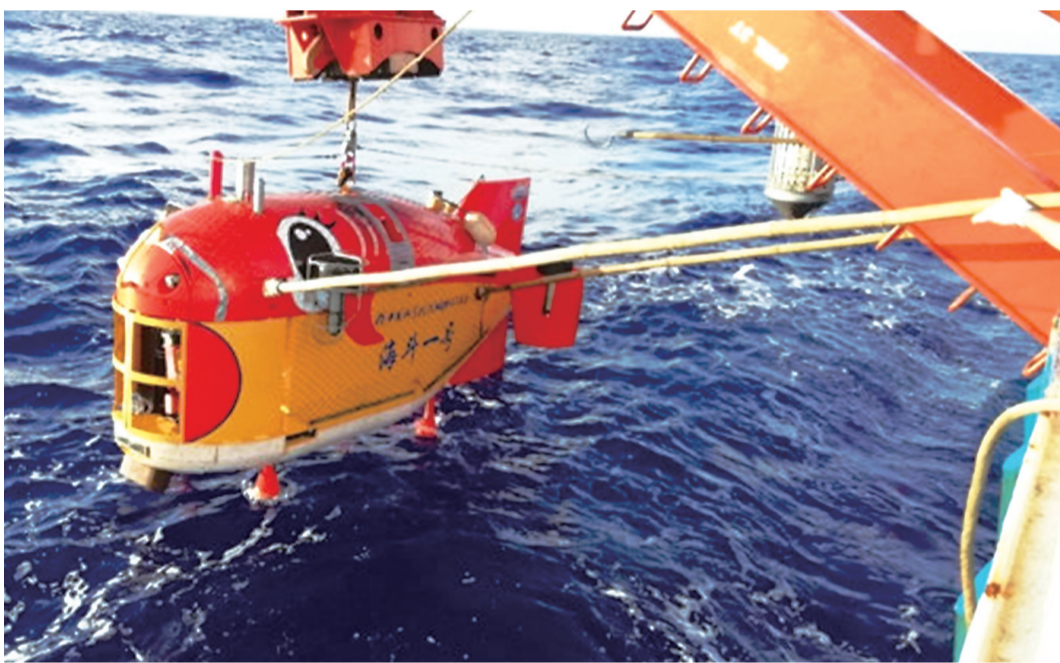
“海斗一号”布放过程。中国科学院沈阳自动化研究所供图
