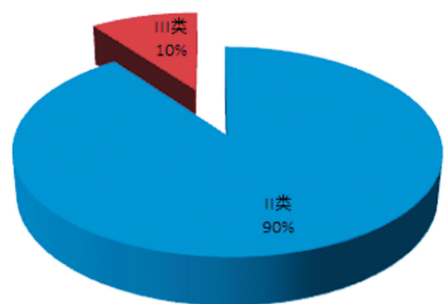
▲2019年江河(湖泊)水系省控以上断面水质类别。
