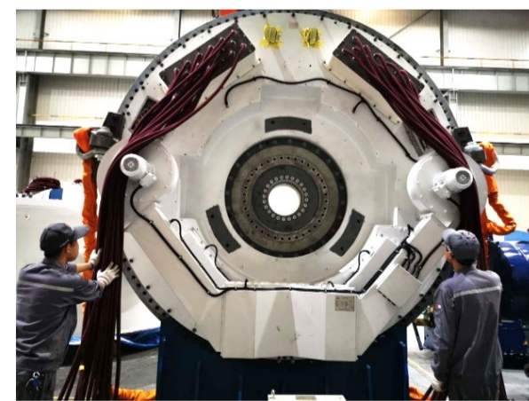
国内首台7MW海上半直驱永磁风力发电机完成组装 通讯员供图
