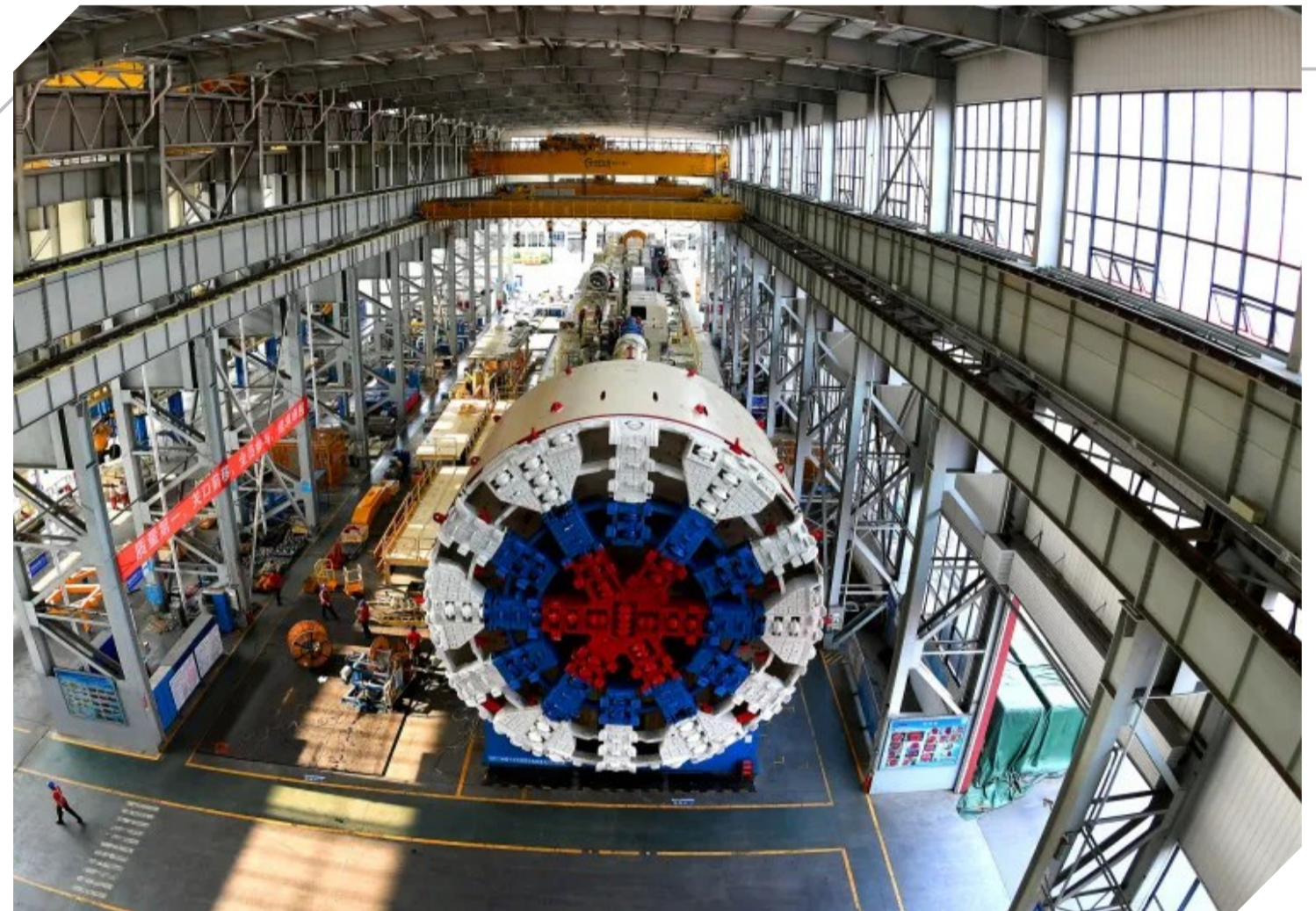
▲出口俄罗斯的11米级大直径盾构机“胜利号”。盾构机是目前用于隧道掘进的先进施工设备 受访企业供图
