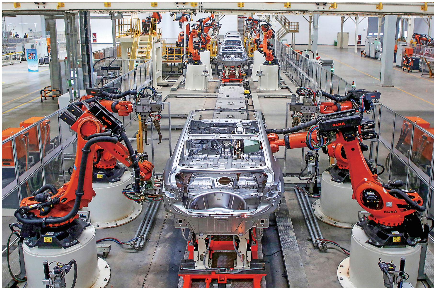
北汽株洲基地二工厂焊装车间,焊接机器人正在工作。
