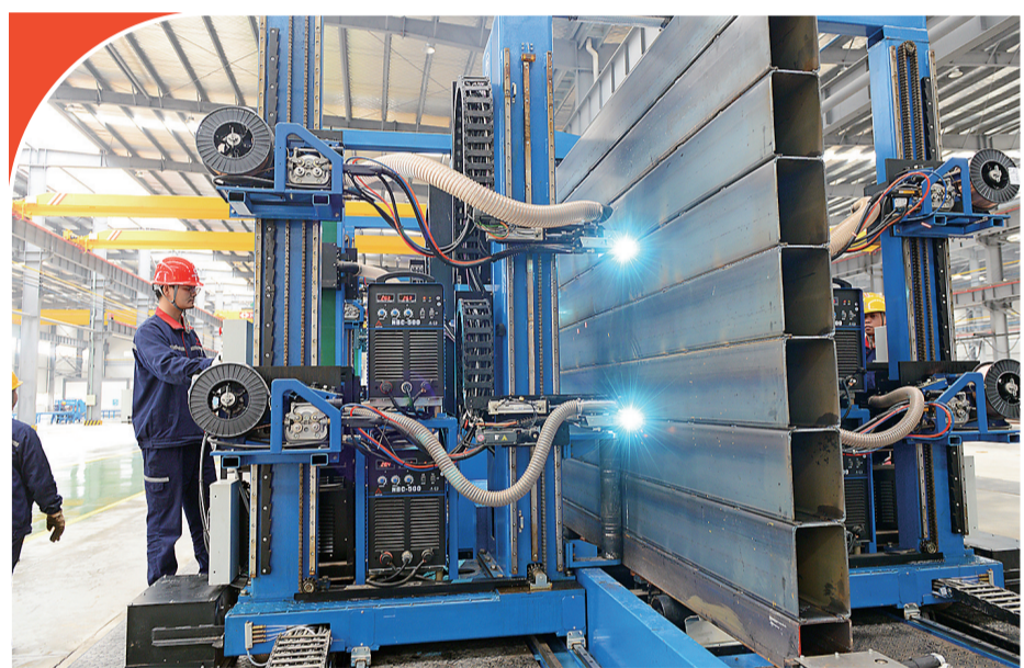
湖南中天杭萧钢构科技股份有限公司株洲生产基地,钢管束焊机正使用激光跟踪焊缝对钢管束构件进行连续焊接。
