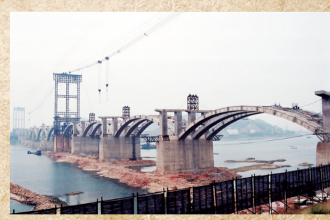
▲石峰大桥正在建设中的情形,其桥身最大跨度为619米,被誉为“神州第一跨”。 陈瑛 摄
