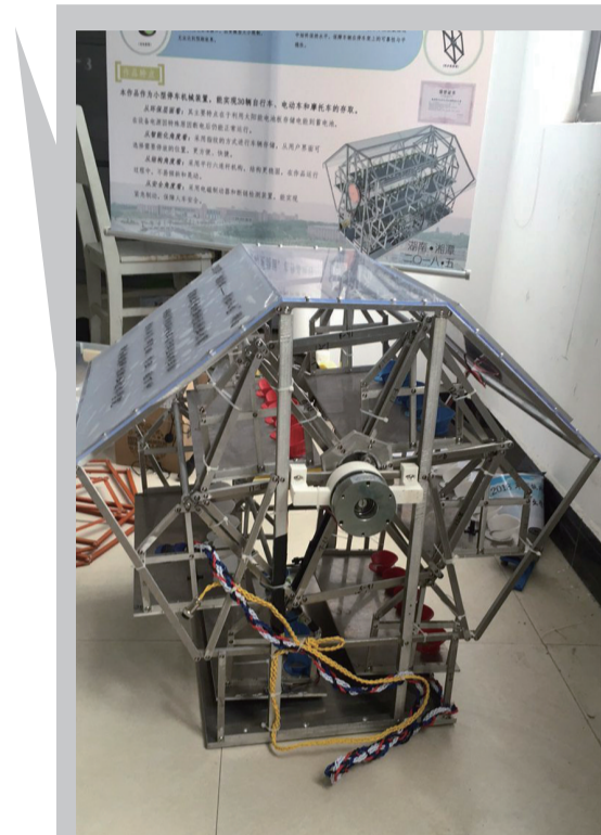
▲旋转式摩托车电动车自行车立体停车库模型
