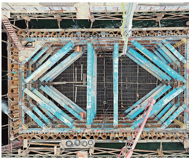
醴娄高速湘江特大桥12号墩浇筑施工现场。通讯员/唐瑞翼 摄
