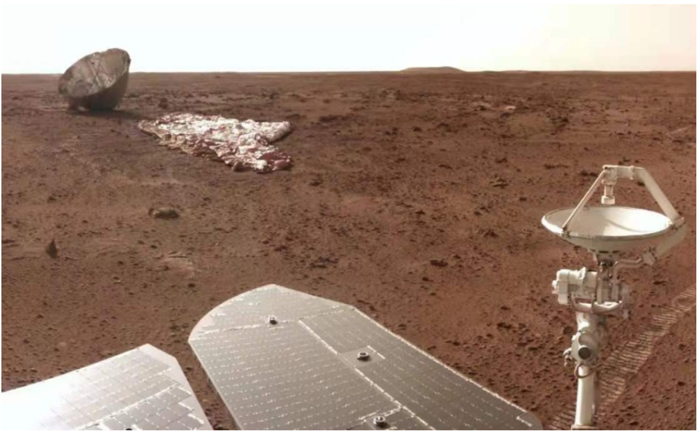
图为降落伞与背罩图像。
